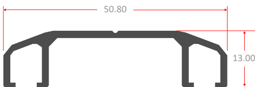
TAPA POLICARBONATO (25-2227)
