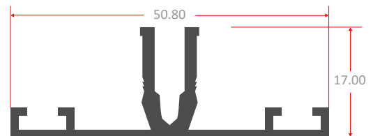
BASE POLICARB. (5-2228)
